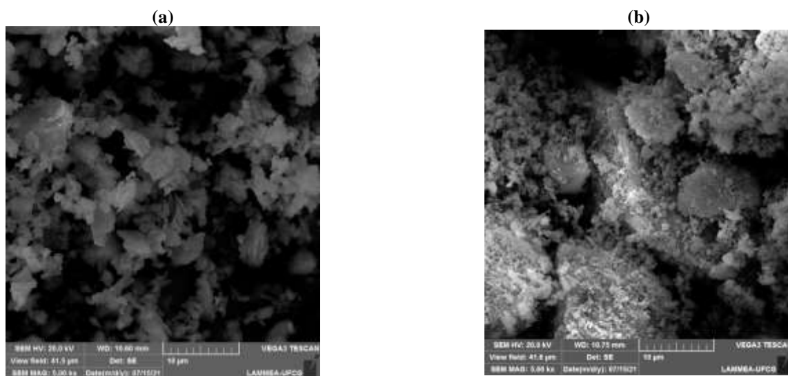
Figura 9 — Micrografias (5000x) dadas por MEV das amostras após tratamento térmico de 1200°C, com taxa de aquecimento de 2°C/min.: (a) caulim comercial; (b) resíduo de caulim.
