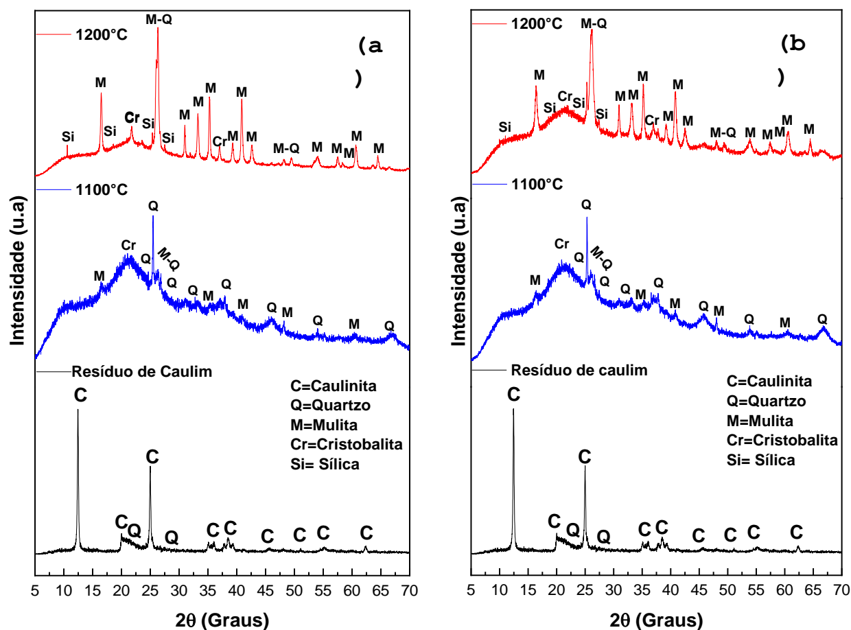
Figura 7 — Difração de raios-X para o resíduo de caulim antes e após tratamento térmico de 1100°C e 1200°C, com taxa de aquecimento de (a) 2°C/min. e (b) 30°C/min.
