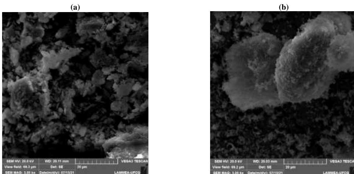
Figura 5 — Micrografias (3000X) para as matérias primas argilosas: (a) caulim comercial (b) resíduo de caulim.
