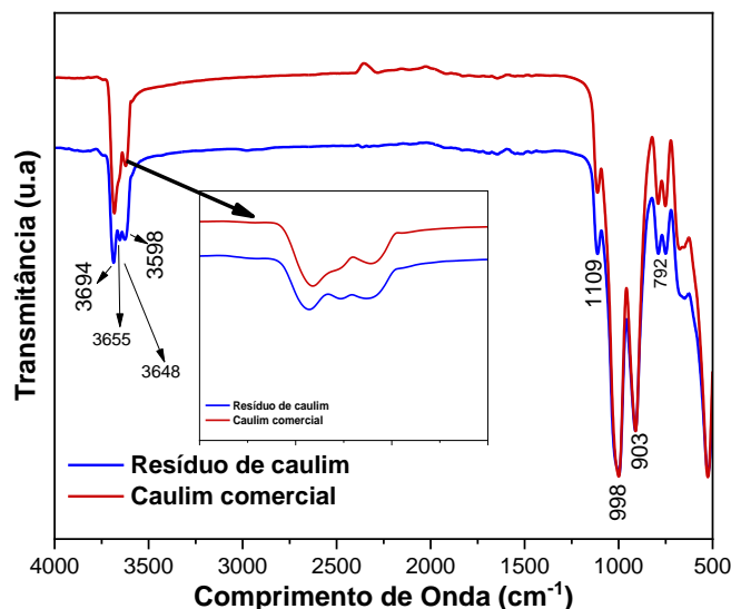
Figura 2 — Espectro na região do infravermelho para os as amostras argilosas de caulim comercial e resíduo de caulim.
