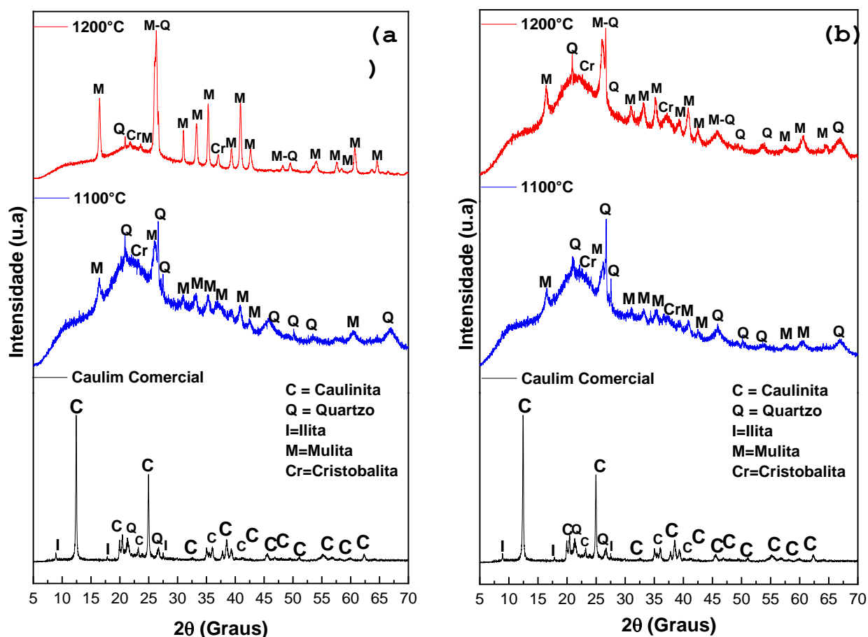
Figura 6 — Difração de raios-X para o caulim comercial antes e após tratamento térmico de 1100°C e 1200°C, com taxa de aquecimento de (a) 2°C/min. e (b) 30°C/min.
