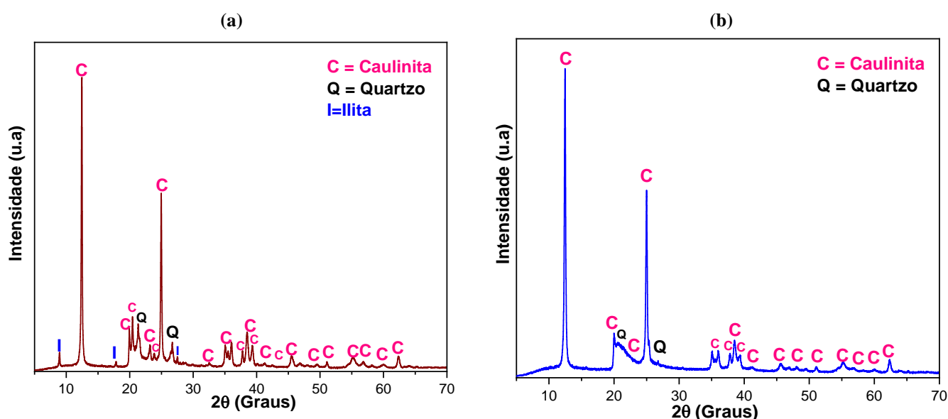
Figura 1 — Difração de raios X das matérias-primas: (a) caulim comercial e (b) resíduo de caulim.
