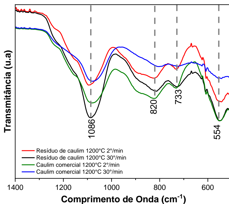
Figura 8 — Espectros vibracionais de FTIR na faixa de 1400 – 500 \text{cm}^{-1} para as amostras de caulim comercial e resíduo de caulim após tratamento térmico de 1100°C e 1200°C, com taxas de 2° e 30°C/min.
