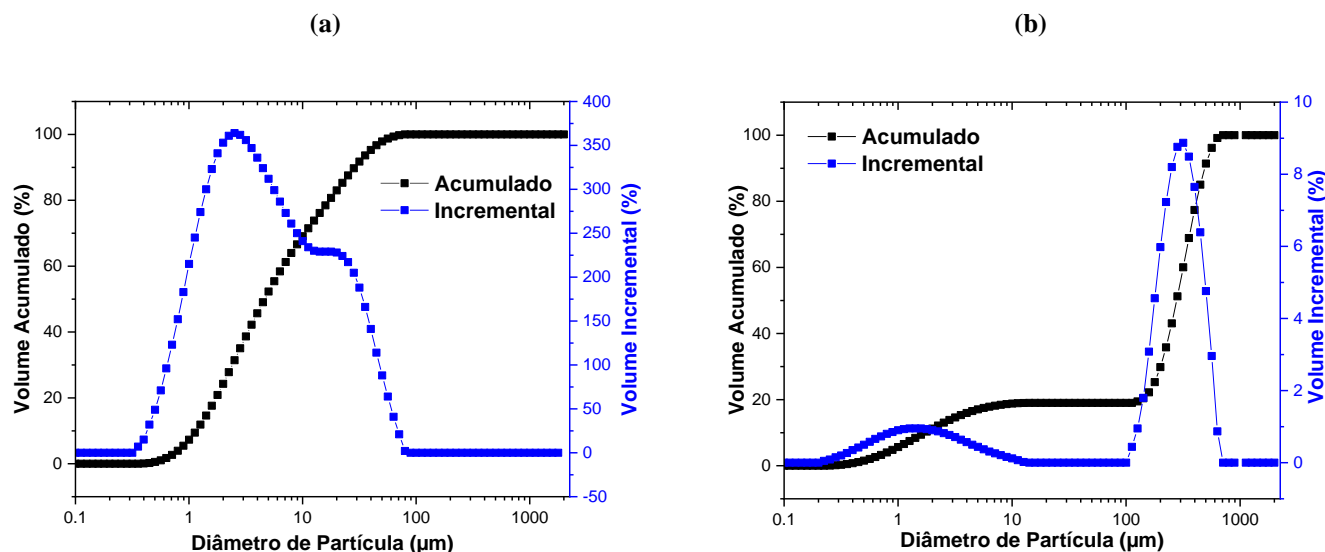
Figura 3 — Distribuição granulométrica das argilas: Caulim (a) e resíduo de caulim (b).
