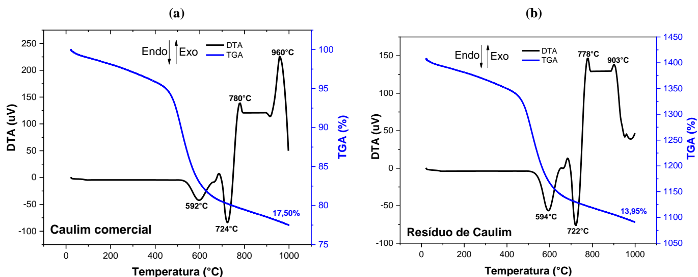
Figura 4 — Curvas de análises térmicas diferenciais (DTA) e termogravimétricas (TGA) das amostras: (a) caulim comercial e (b) resíduo de caulim.
