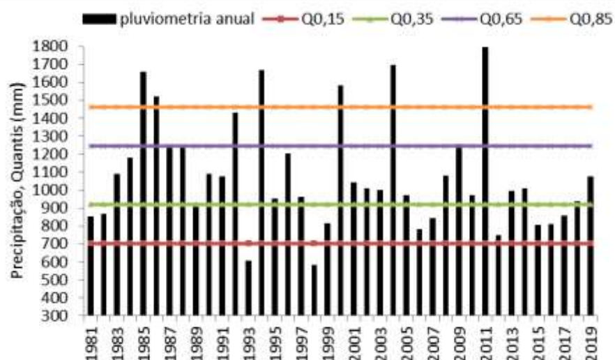
Figura 2. Distribuição pluvial anual e seus valores quantis Q_{(0,15)} , Q_{(0,35)} , Q_{(0,65)} e Q_{(0,85)} , para o município de Lagoa Seca - PB.
