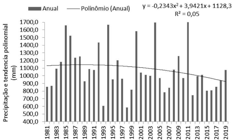
Figura 3 - Precipitação anual (mm) e sua reta de tendência polinomial, para o período de 1981-2019 no município de Lagoa Seca - PB.
