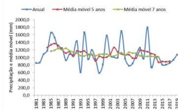
Figura 5 - Precipitação anual e suas retas de tendência média móvel para 5 e 7 anos no período de 1981-2019 em Lagoa Seca - PB.
