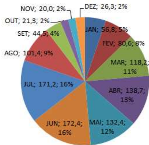
Figura 4 – Distribuição da precipitação mensal (mm) e seus valores percentuais no período de 1981-2019 no município de Lagoa Seca - PB.
