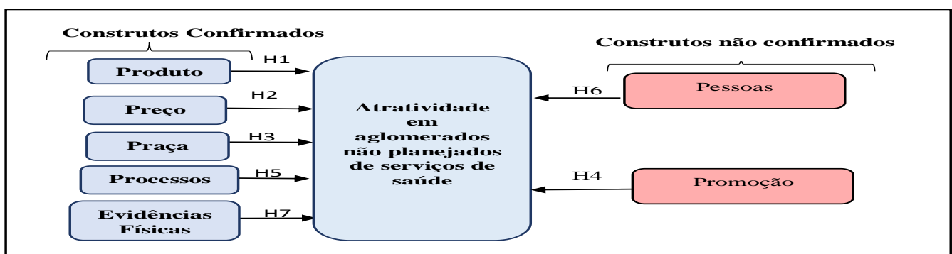
Figura 4. Resultado da Pesquisa.
