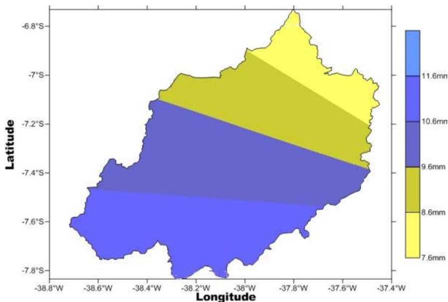
Figura 16. Isoieta do período seco na BHRPB.
