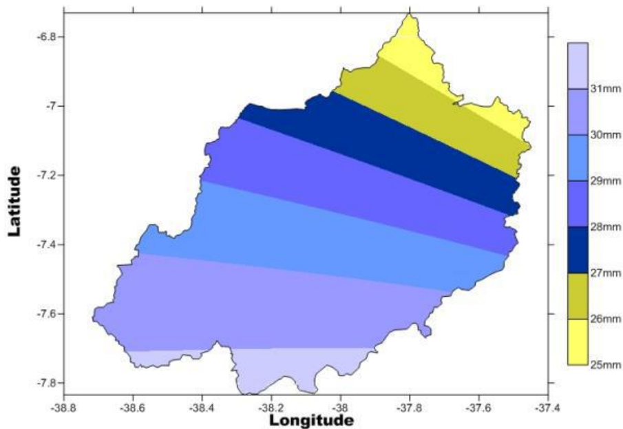
Figura 15. Isoieta do período chuvoso na BHRPB.
