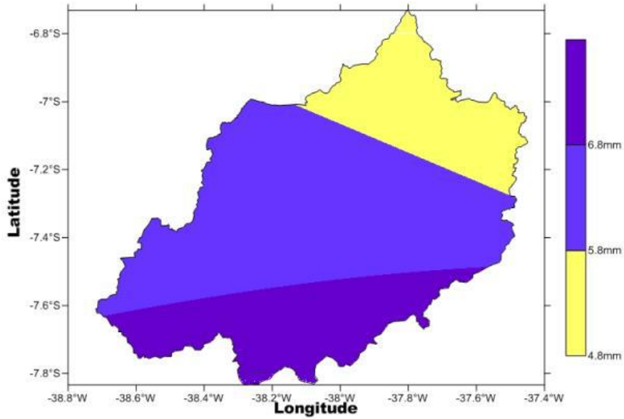
Figura 11. Isoieta do mês de outubro na BHRPB.
