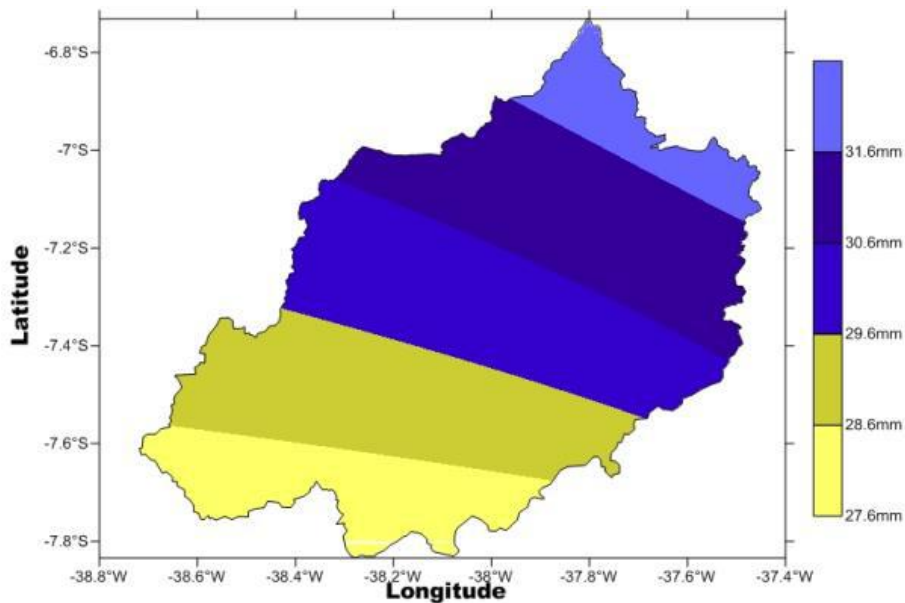
Figura 9. Isoieta do mês de agosto na BHRPB.
