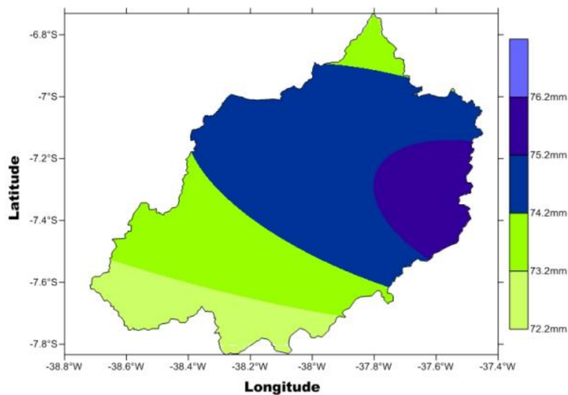
Figura 6. Isoieta do mês de maio na BHRPB.
