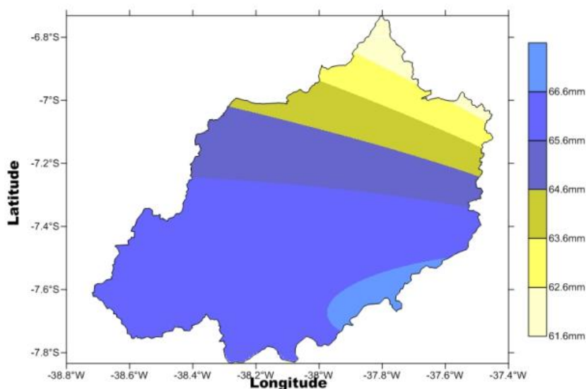
Figura 2. Isoieta do mês de janeiro na BHRPB.
