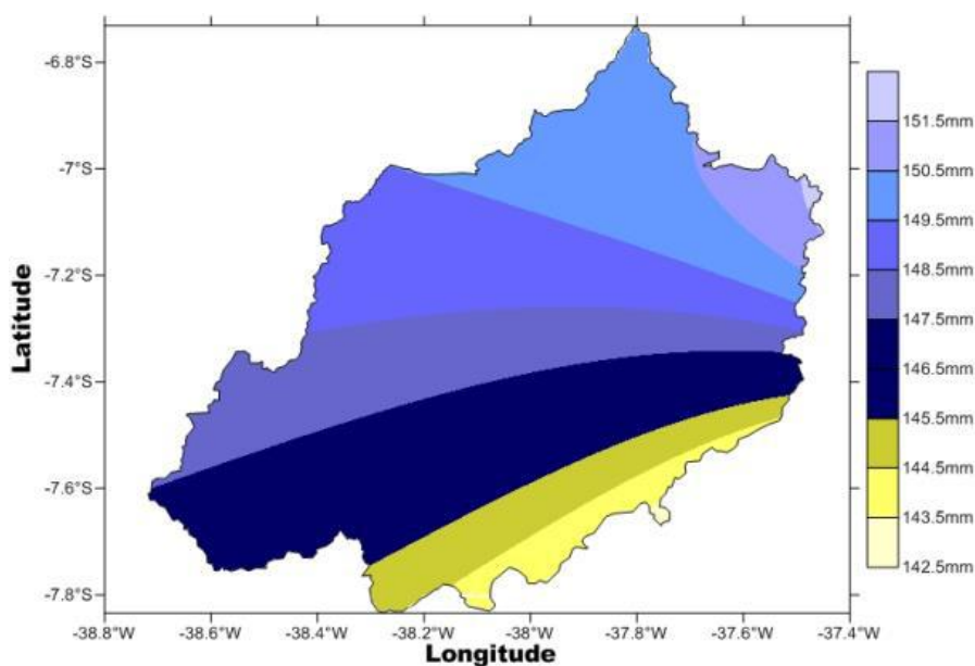
Figura 4. Isoieta do mês de março na BHRPB.
