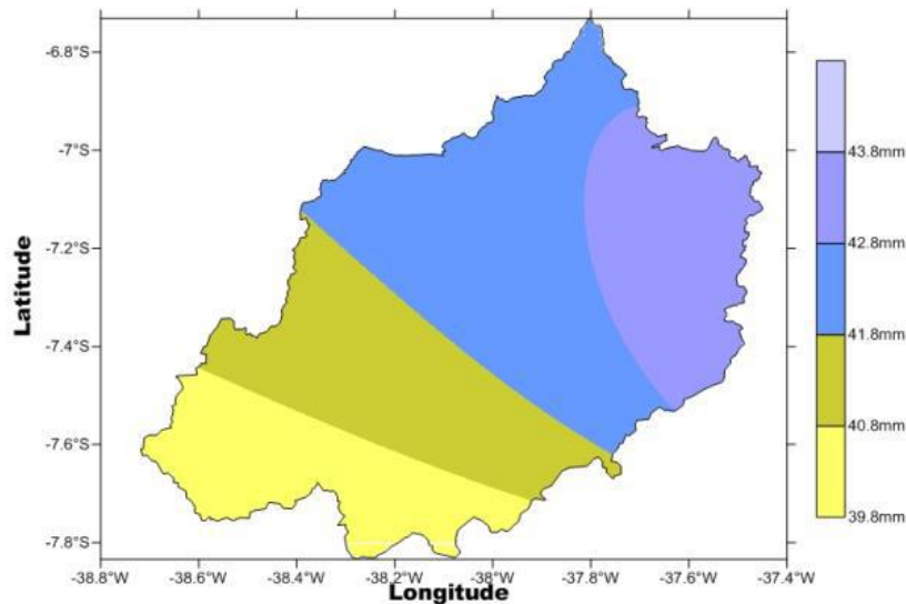
Figura 8. Isoieta do mês de julho na BHRPB.
