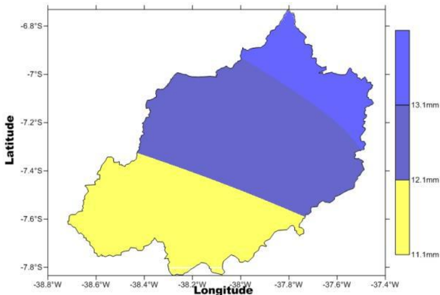
Figura 10. Isoieta do mês de setembro na BHRPB.
