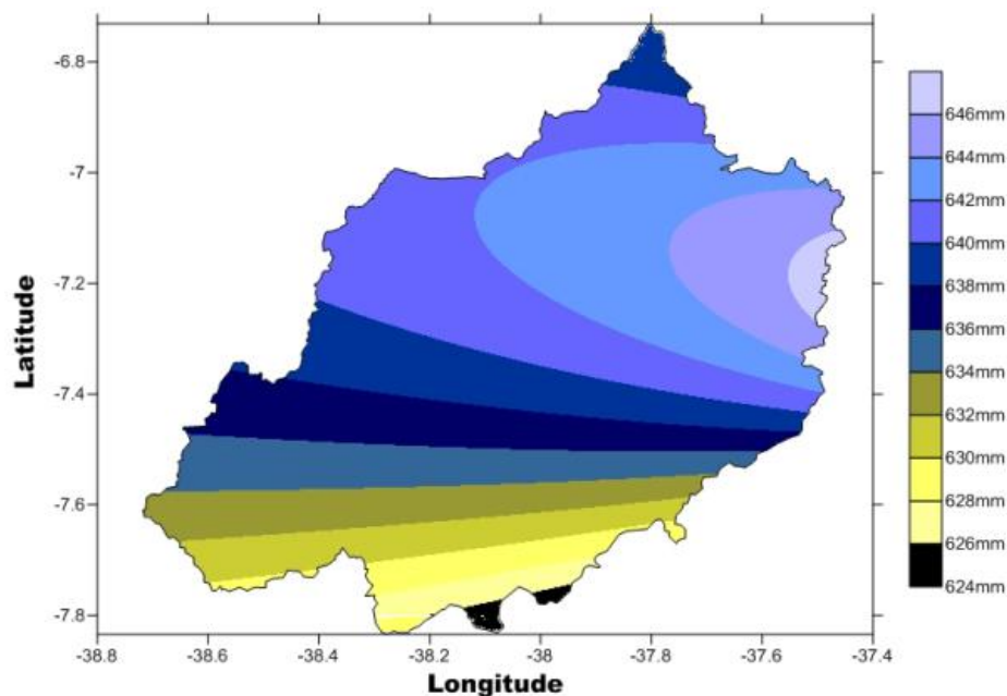
Figura 14. Isoieta anual na BHRPB.
