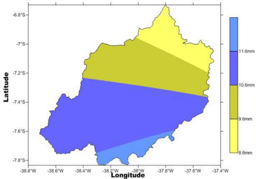
Figura 12. Isoieta do mês de novembro na BHRPB.
