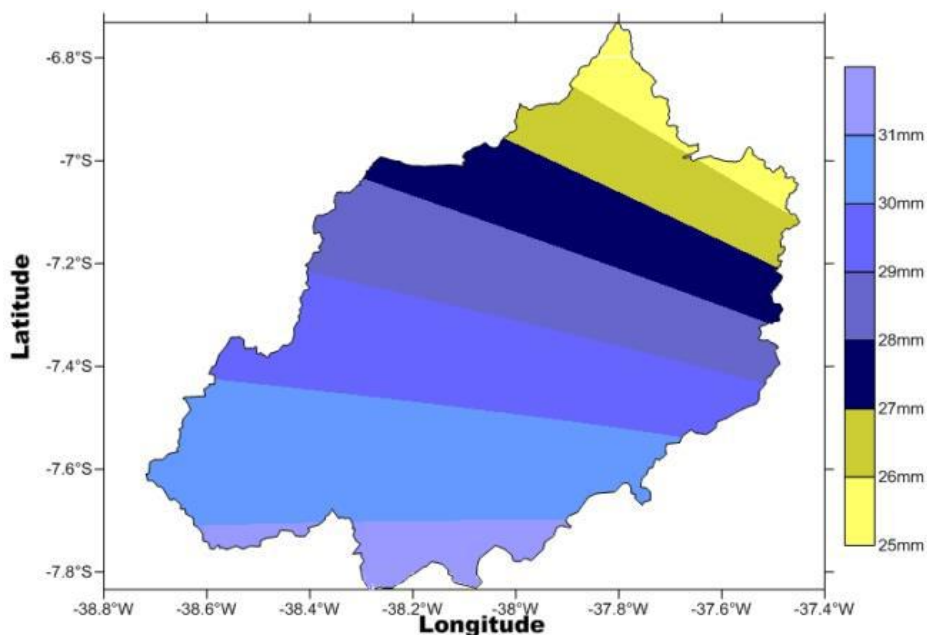
Figura 13. Isoieta do mês de dezembro na BHRPB.
