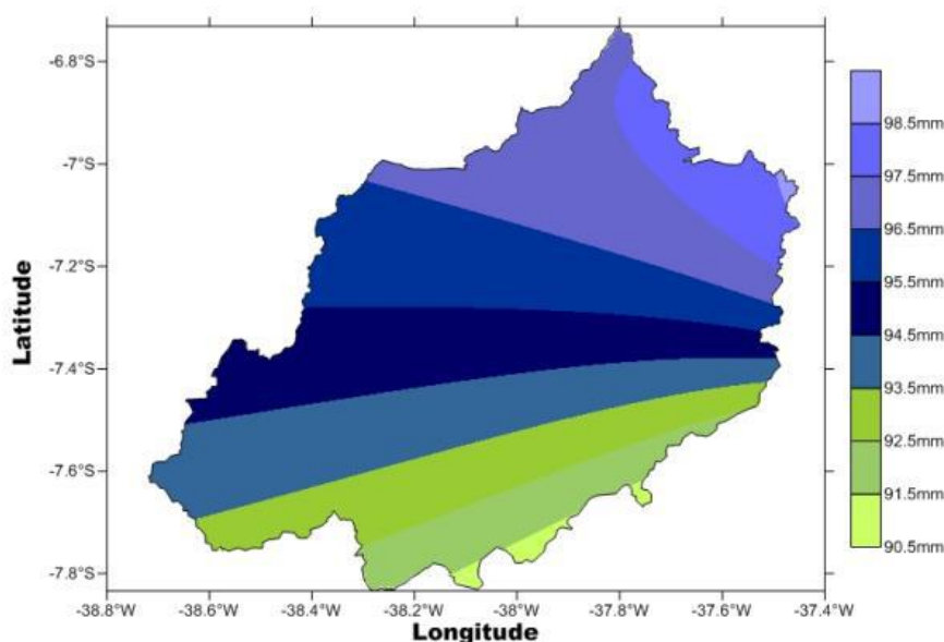
Figura 3. Isoieta do mês de fevereiro na BHRPB.
