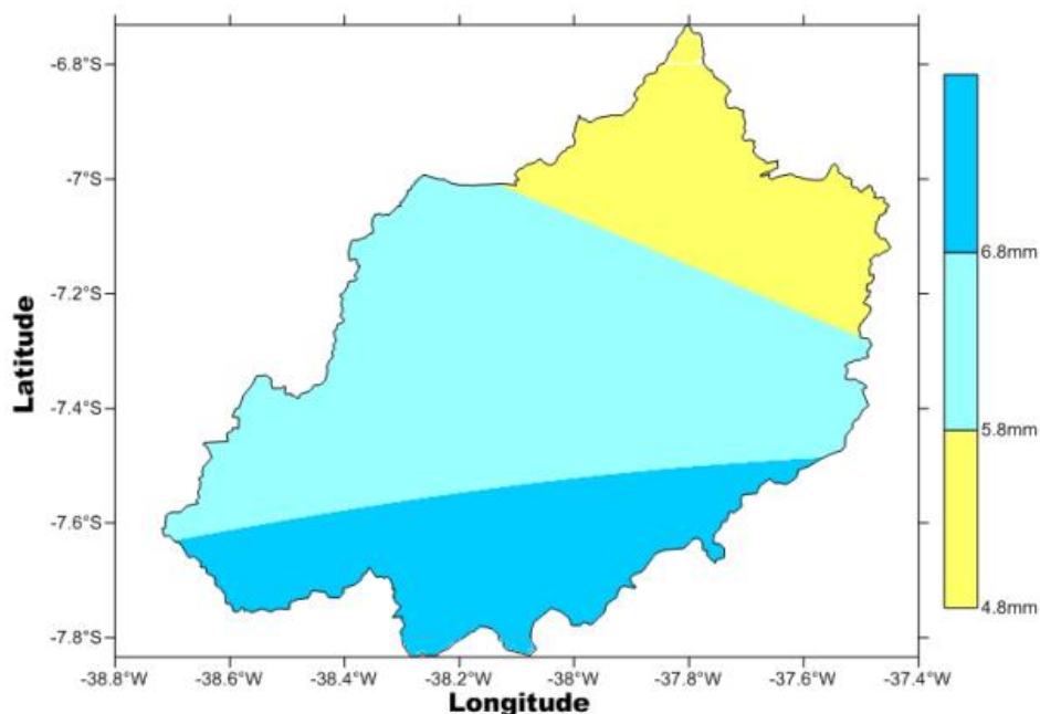
Figura 20. Isoieta do mês seco na BHRPB.
